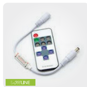
دیمر ۲۴~۱۲ ولت ۱۲ آمپر با کنترلر RF برای ریسرهای LowLine
